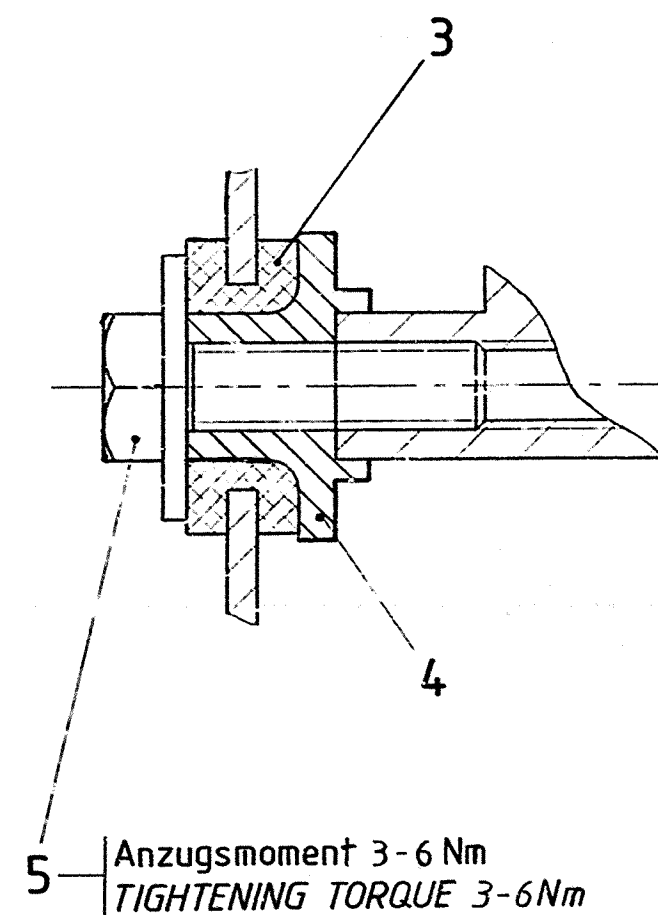
Einzelheit Z M 2:1
